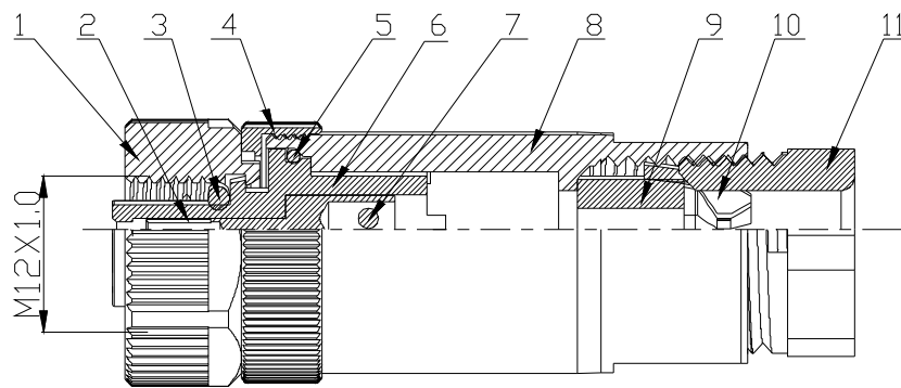
截面 A-A
