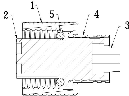
截面 A-A
