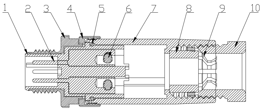
截面 A-A
