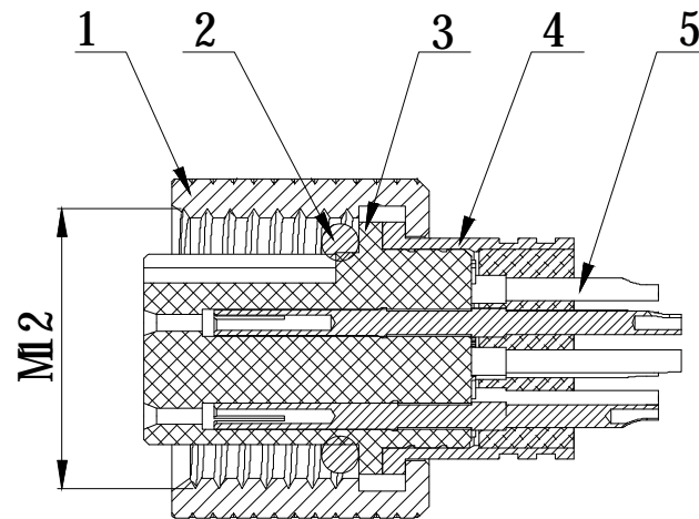
截面 A-A
