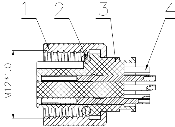
截面 A-A
