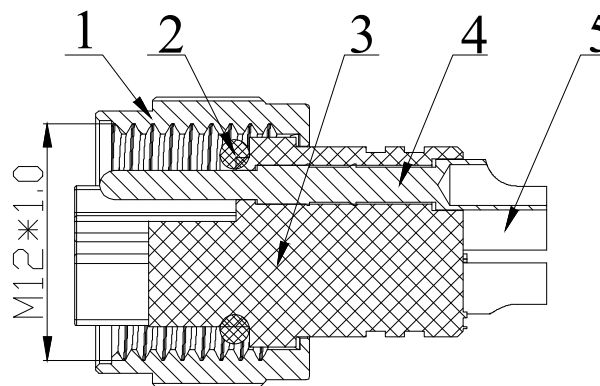
截面A-A
