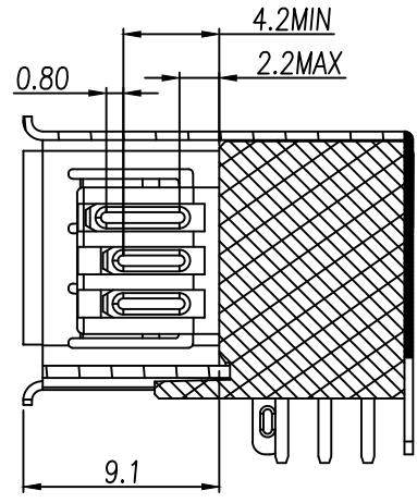
截面 A-A
