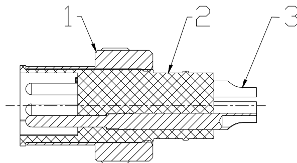
截面A-A
