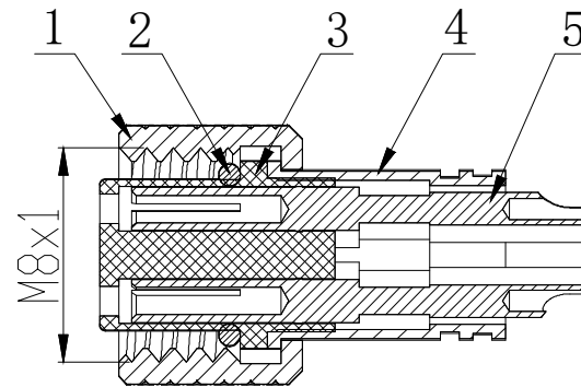
截面A-A
