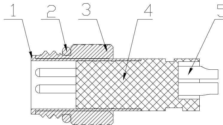
截面A-A
