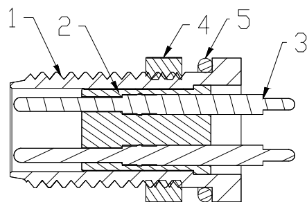
截面 A-A
