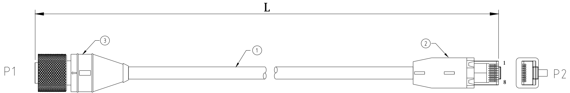
M12 5P母 D扣带屏蔽焊成型式
